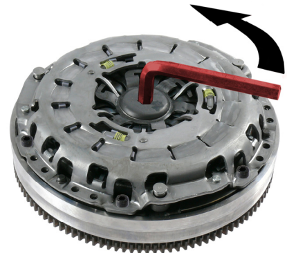
Abb./Fig. 3: Verriegelungsstück herausdrehen / Unscrew locking piece / Retirer la pièce de verrouillage en tournant / Desenroscar la pieza de enclavamiento / Rimozione dell'elemento di bloccaggio
